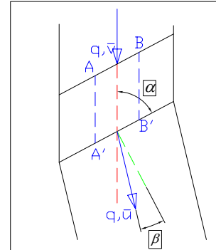
Figura N° 3. Vertedero oblicuo en un canal
