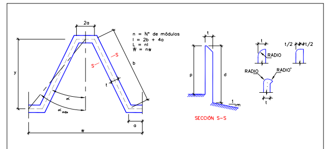
Figura N° 2. Aliviadero tipo laberinto. Definición geométrica
