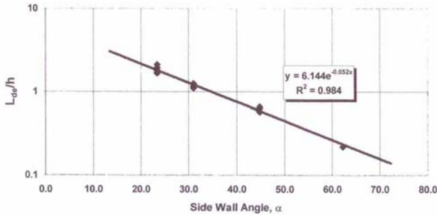
Figura N° 5. Indlekofer y Rouve, 1975. Relación L_{de} - \alpha
