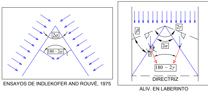
Figura N° 6. Interferencia de láminas en vertederos en laberinto
