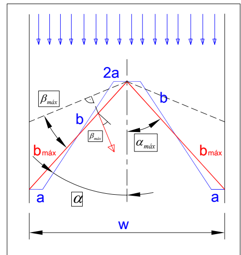
Figura N° 7. Interferencia de láminas. Simplificación para vertederos trapeziales
