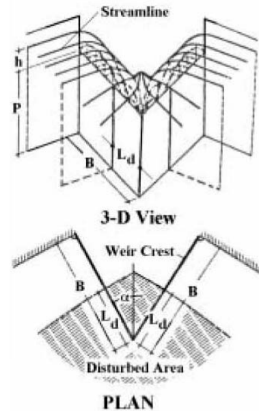
Figura N° 4. Indlekofer y Rouve, 1975. Interferencia de láminas
